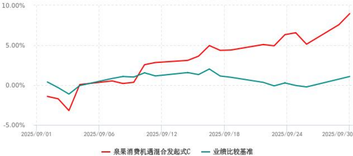
泉果消费机遇混合发起式C累计净值增长率与业绩比较基准收益率历史走势对比图 (2025年09月01日-2025年09月30日)
